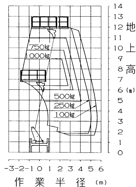
アウトリガ最小張出
